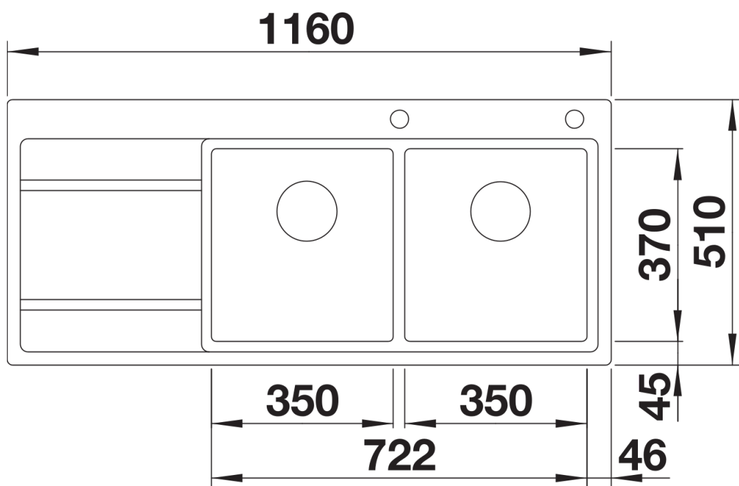
Bovenaanzicht
