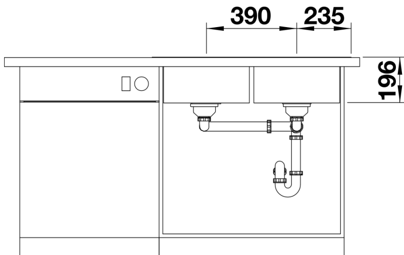
Vooraanzicht
