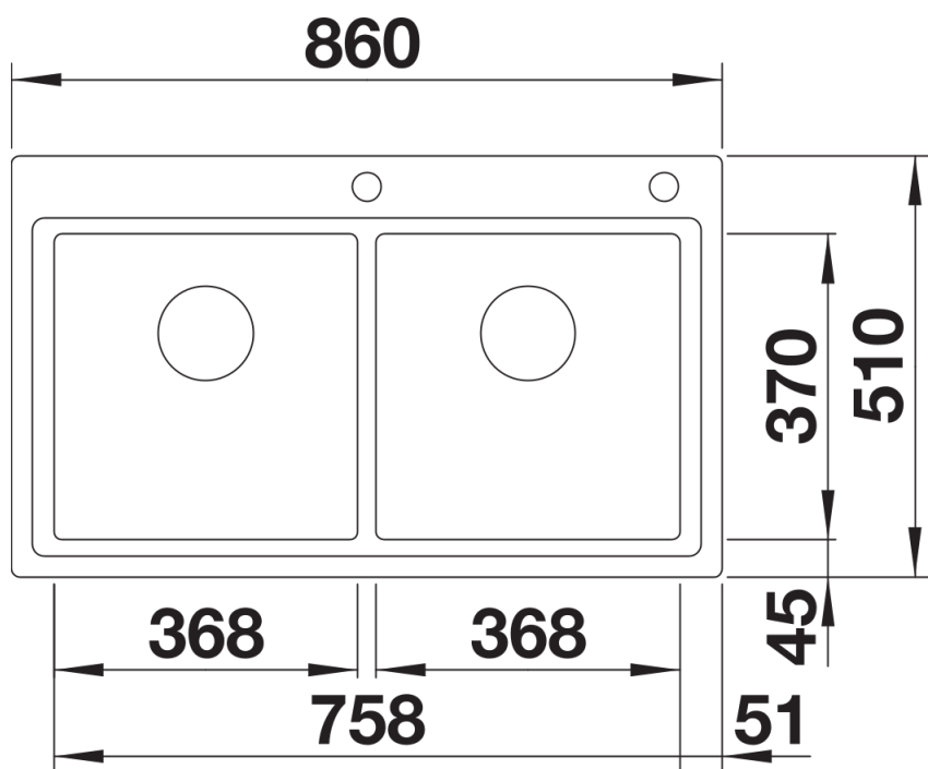
Bovenaanzicht
