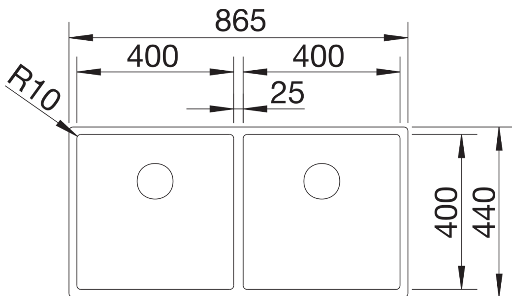
Bovenaanzicht
