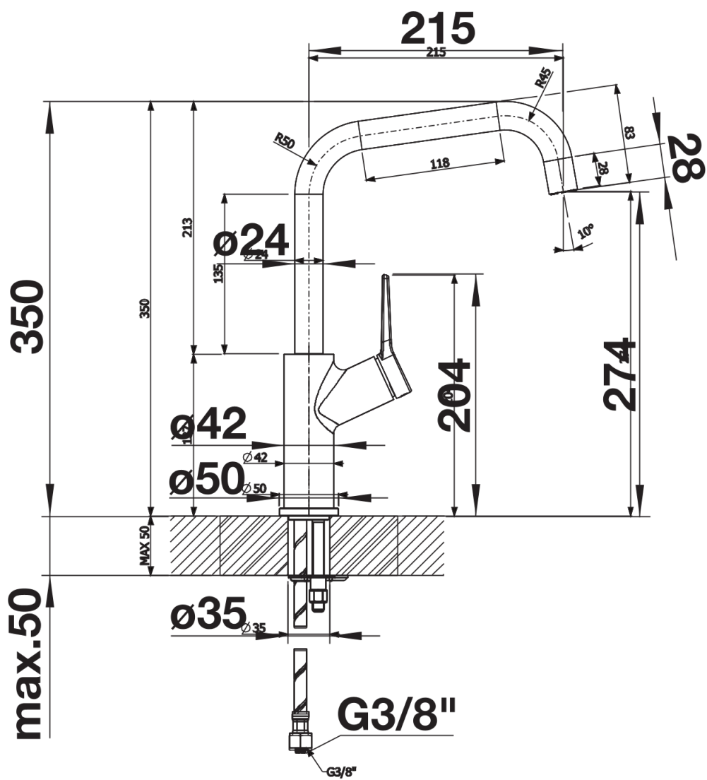
Vue latérale
