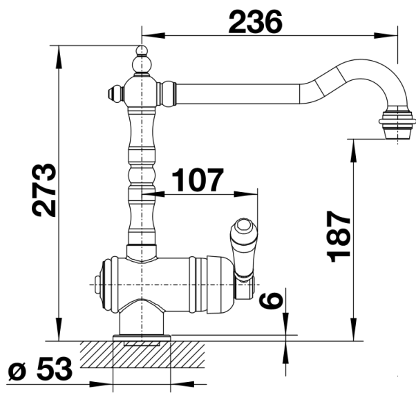
Zijaanzicht
