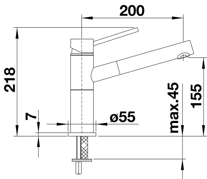
Zijaanzicht
