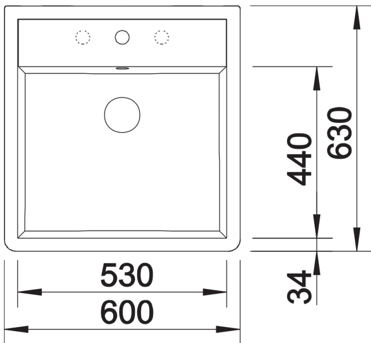
Bovenaanzicht
