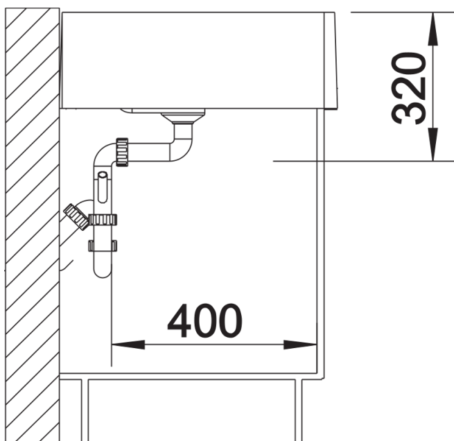
Zijaanzicht
