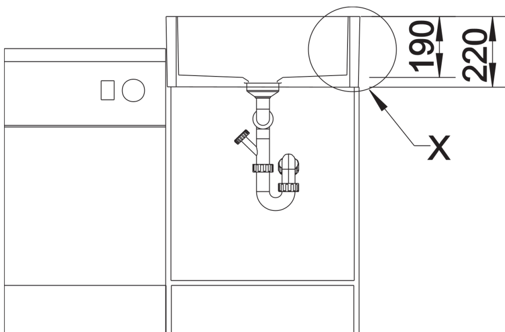
Vooraanzicht
