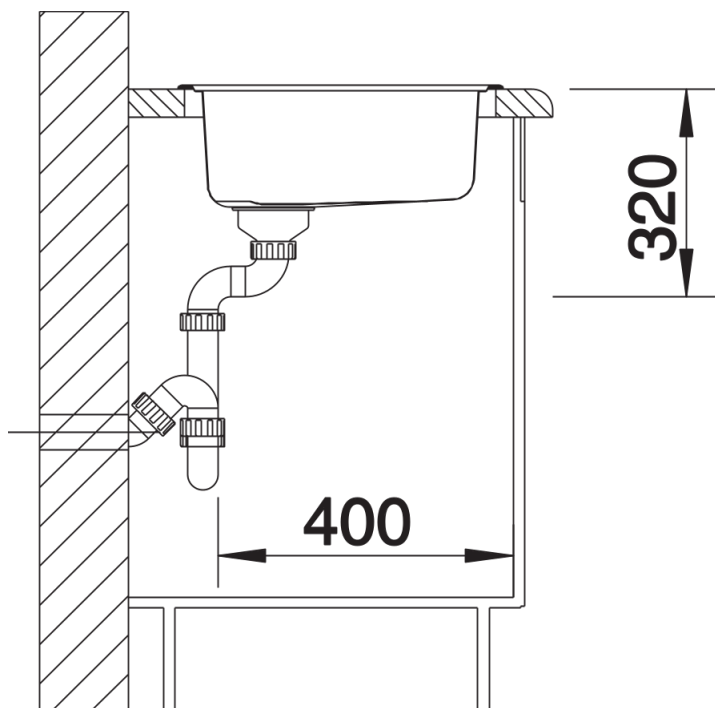
Zijaanzicht
