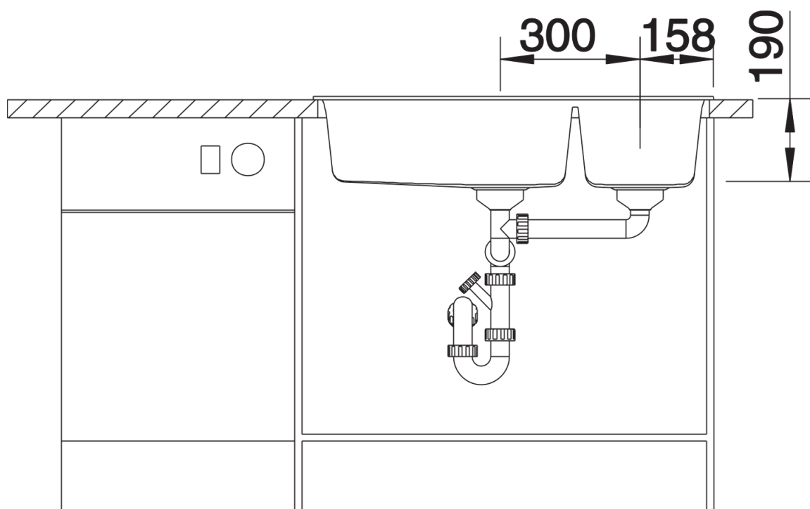
Vooraanzicht
